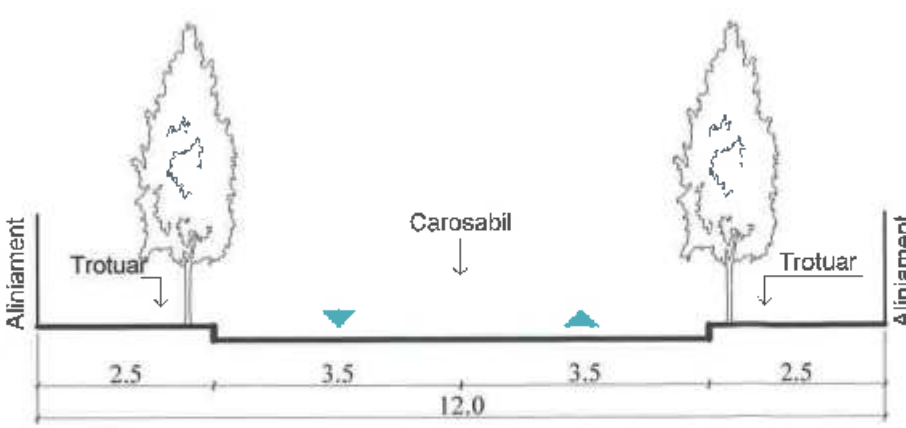
Profil stradal existent si propus Strada Salajeni
